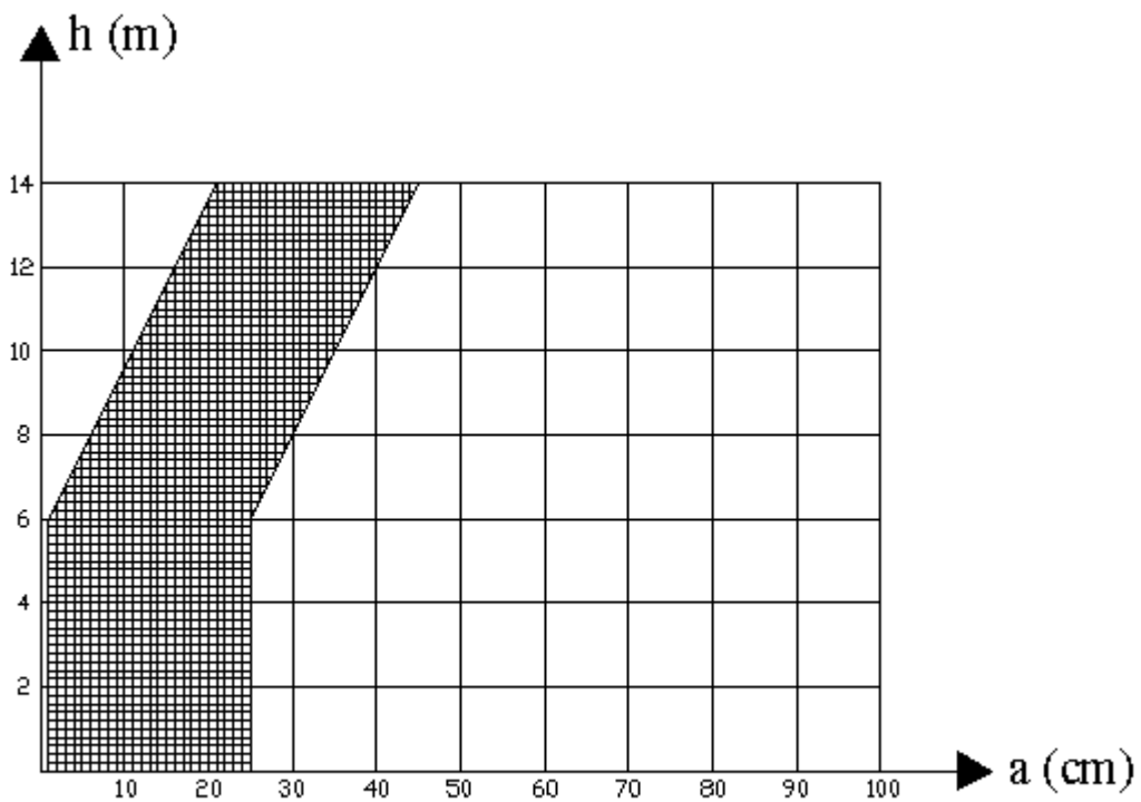
Takhelling opp til 1:5 ( 11^\circ )
