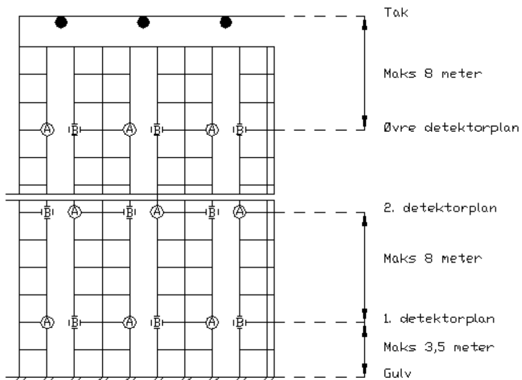
Figur 10 Vertikalt tverrsnitt
